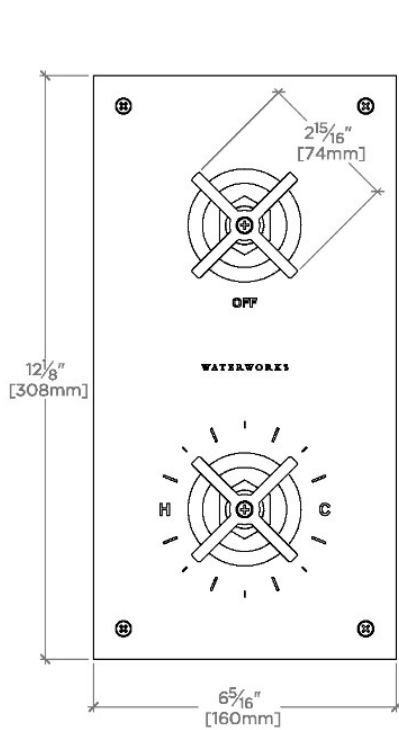
FRONT VIEW SCALE: 3"=1'-0"
