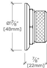
SIDE VIEW SCALE: 6"=1'-0"
