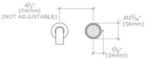
TOP VIEW SCALE: 1\frac{1}{2}"=1'-0"
