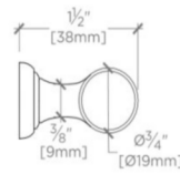
SIDE VIEW SCALE: 6"=1'-0"
