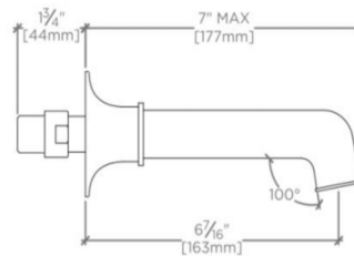
SIDE VIEW SCALE: 3"=1'-0"
