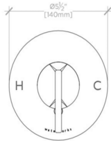
TOP VIEW SCALE: 3"=1'-0"
